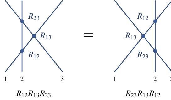
Şekil 8.2 Kuantum Yang–Baxter denkleminin doğru-diyagramı. Üç doğru ikişerli kesişir; her kesişim bir R_{ij} operatörüdür. İkinci doğruyu R_{13} kesişiminin soluna ya da sağına kaydırmak operatörü değiştirmez: R_{12}R_{13}R_{23} = R_{23}R_{13}R_{12} .
