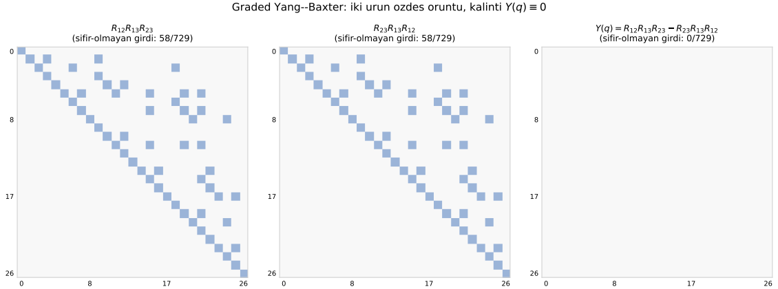
Şekil 9.4 Graded Yang–Baxter denkleminin iki tarafının 27 \times 27 sıfır-olmayan örüntüleri özdeşdir; kalıntı Y(q) = R_{12}R_{13}R_{23} - R_{23}R_{13}R_{12} tüm 729 girdide sıfırdır (graded_yang_baxter_residual_GLq21).
